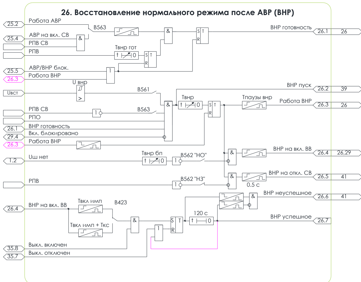
Рисунок 5.24 – Схема №26. Алгоритм ВНР
