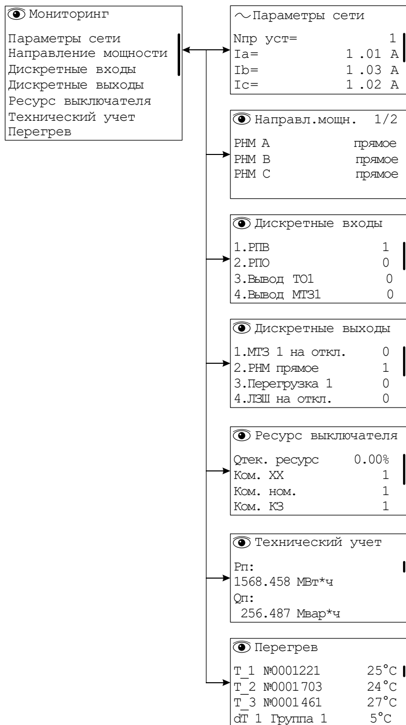
Рисунок 6.8 – Структура раздела «Мониторинг»
