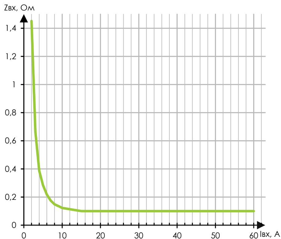
Рисунок 3.1 – Полное сопротивление токового входа блока при отсутствии нагрузки на встроенный источник питания дискретных входов, разомкнутых дискретных выходах, несрабатанном состоянии модуля дешунтирования
