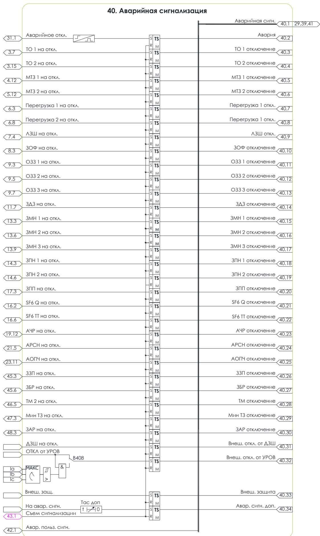
Рисунок 5.41 – Схема №40. Алгоритм аварийной сигнализации
