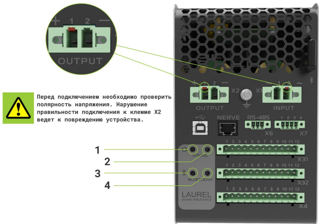
Рисунок 5.3 – Лицевая панель LAUREL
