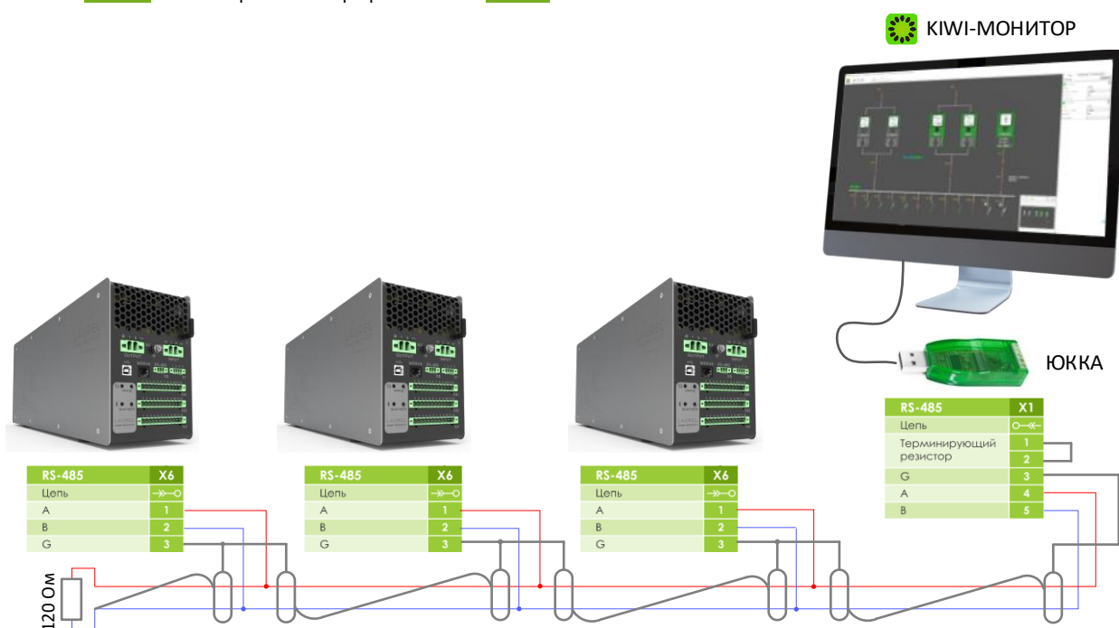
Рисунок П4.15.10 – Схема подключения LAUREL к ПТК KIWI-MONITOR по интерфейсу RS-485
