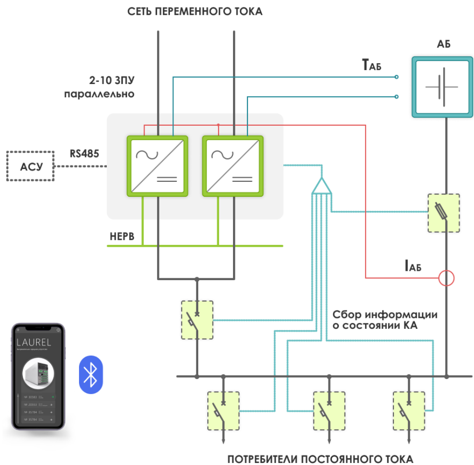
Рисунок П4.15.3 – Структура СОПТ с параллельной работой 3ПУ
