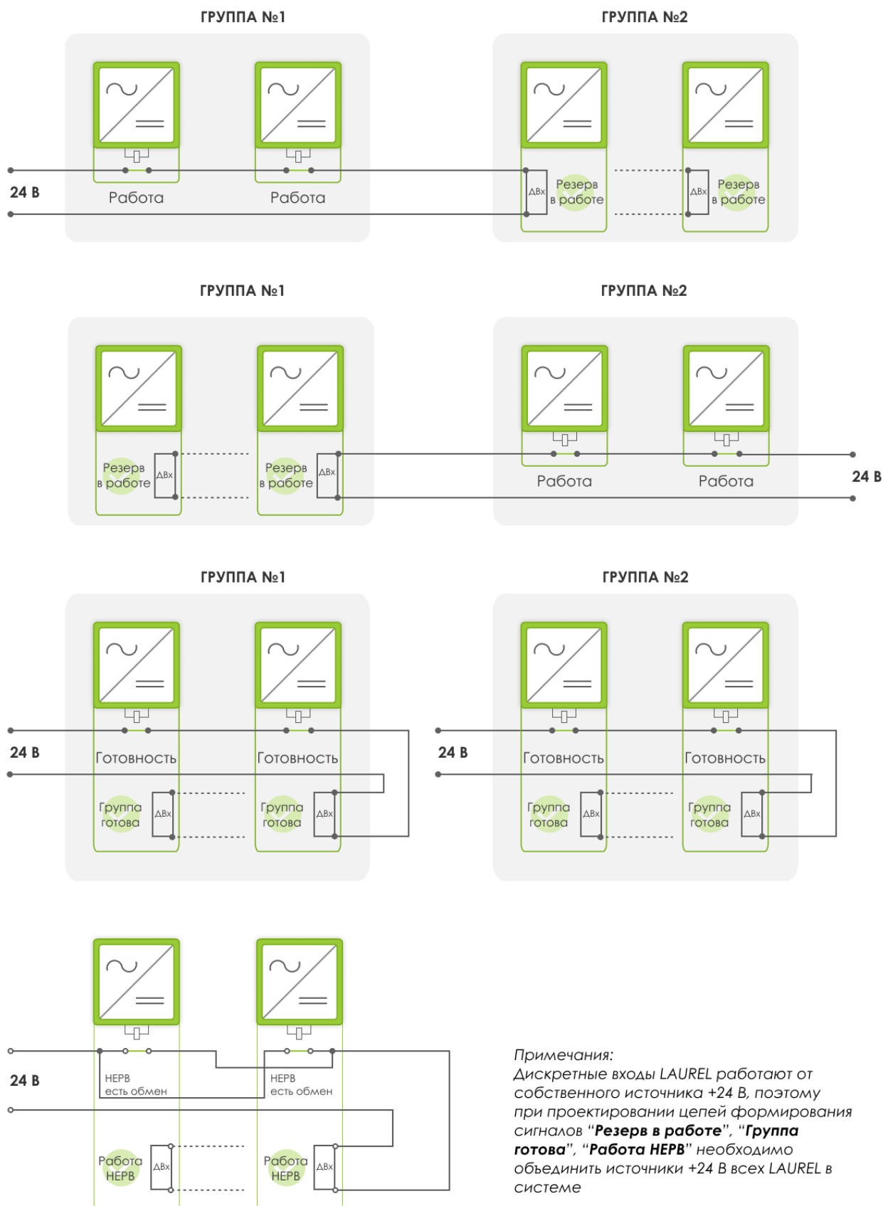
Рисунок П4.15.9 – Схемы подключения дискретных цепей между LAUREL
