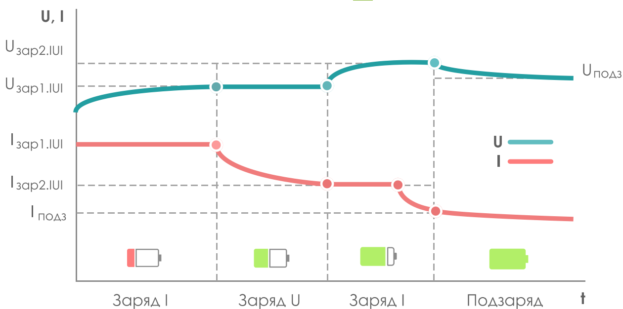
Рисунок 7.8 – График заряда АБ методом IUI
