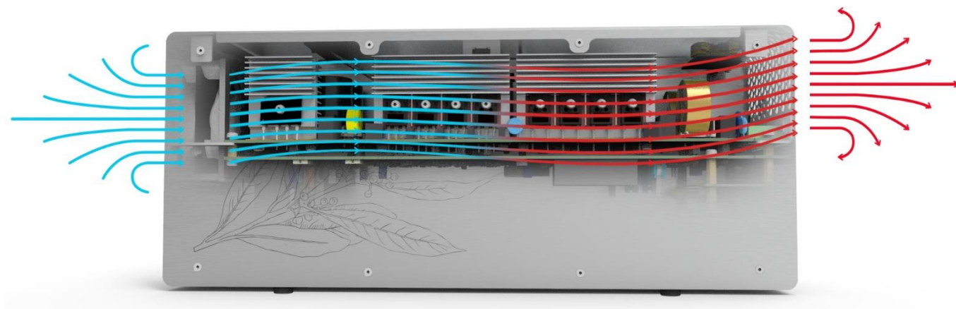
Рисунок 5.2 – Направление воздушного потока при охлаждении LAUREL
