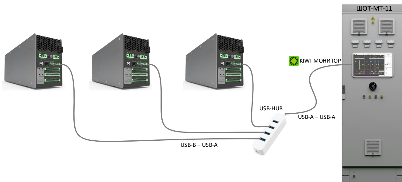
Рисунок П4.15.11 – Схема подключения LAUREL к ПТК KIWI-MONITOR по интерфейсу USB в шкафу оперативного тока
