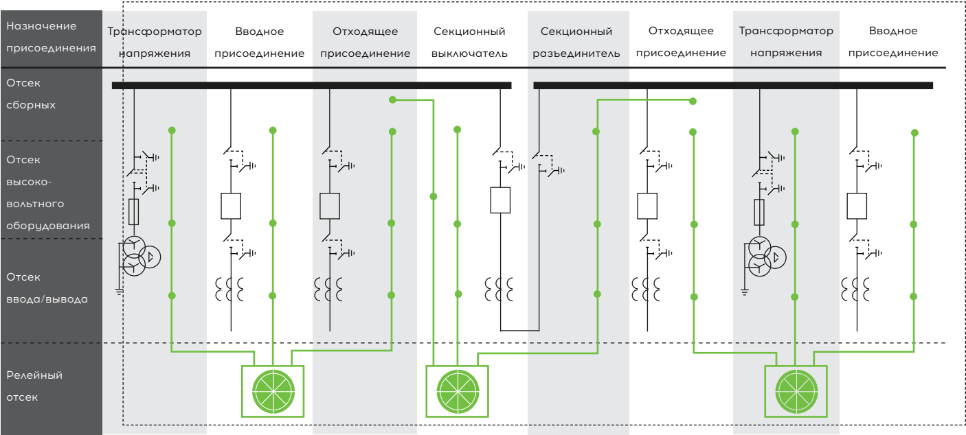
Пример размещение датчиков ТЕКИЛА в ячейках KCO
