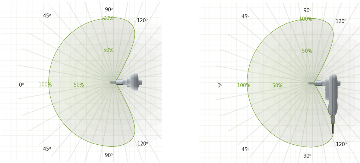
Диаграмма направленности датчика типа ВОД
