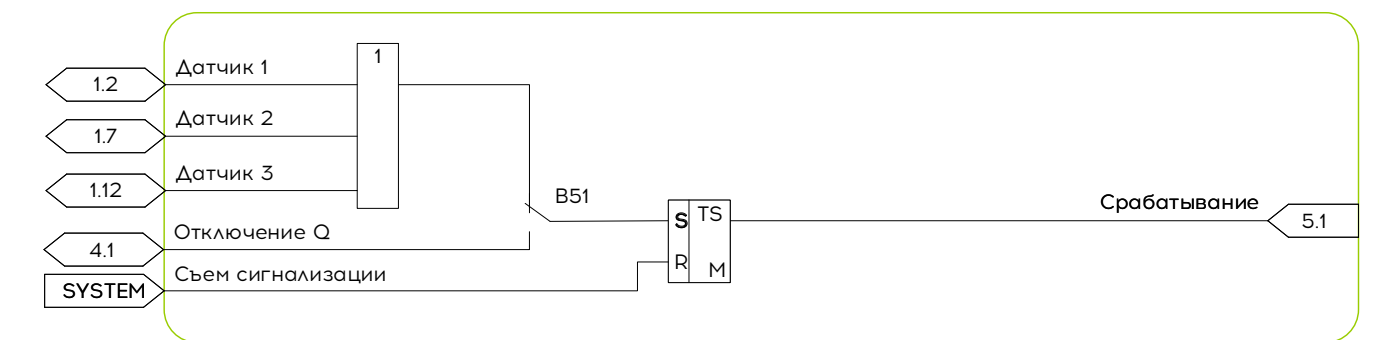
Функциональная схема алгоритма №5 «Сигнализация»
