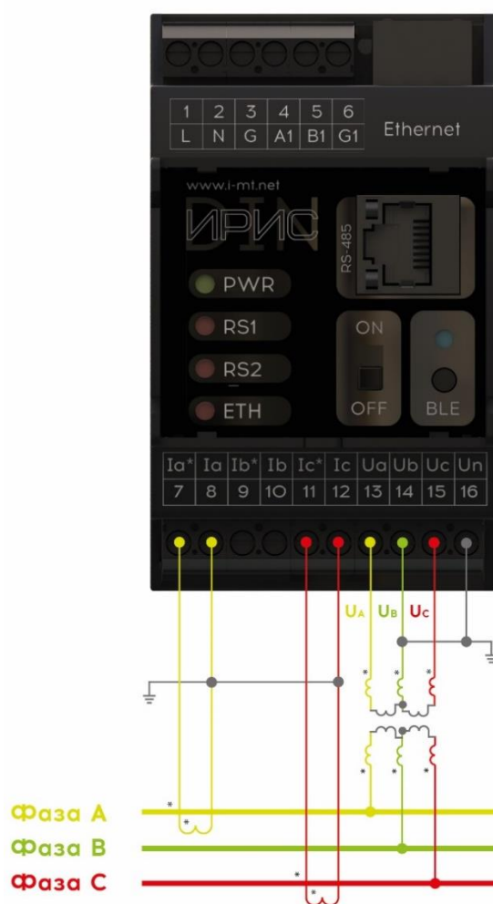
Рисунок 10.5 - Схема подключения устройства с внешними трансформаторами тока и трансформаторами напряжения (2ТТ, 2ТН)
