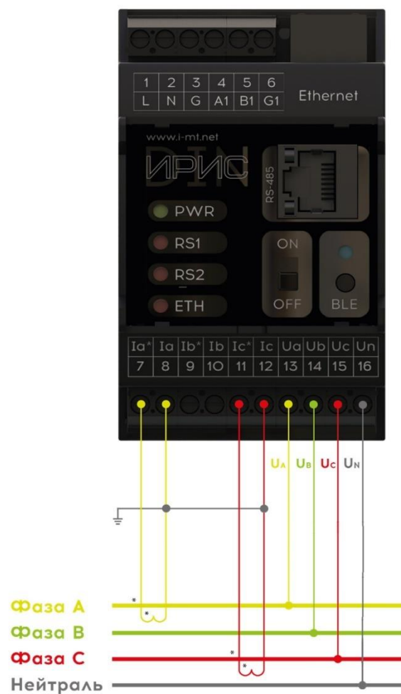
Рисунок 10.4 - Схема подключения устройства с внешними трансформаторами тока, без трансформаторов напряжения (2ТТ, 0ТН)
