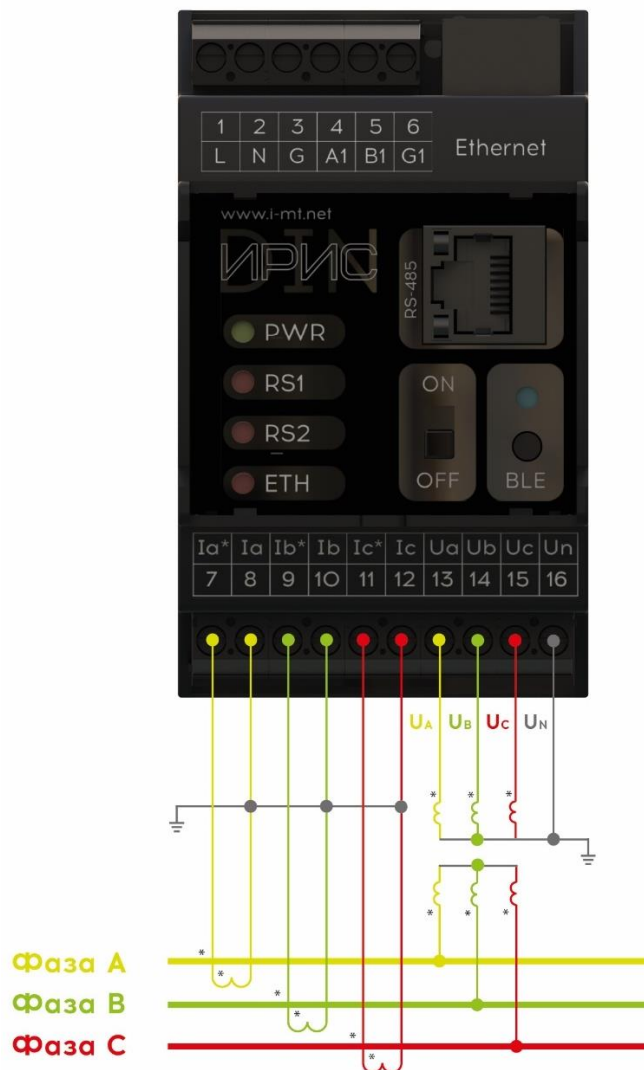
Рисунок 10.2 - Схема подключения устройства с внешними трансформаторами тока и трансформаторами напряжения (ЗТТ, ЗТН)
