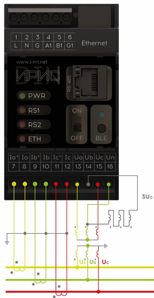
Рисунок 10.6 - Схема подключения устройства с внешними трансформаторами тока и трансформаторами напряжения с дополнительной обмоткой (3ТТ, 3ТНД)
