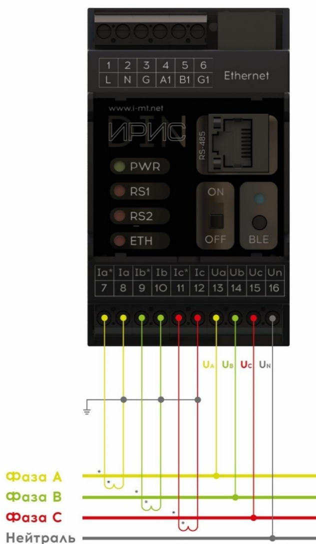
Рисунок 10.1 - Схема подключения устройства с внешними трансформаторами тока, без трансформаторов напряжения (ЗТТ, 0ТН)
