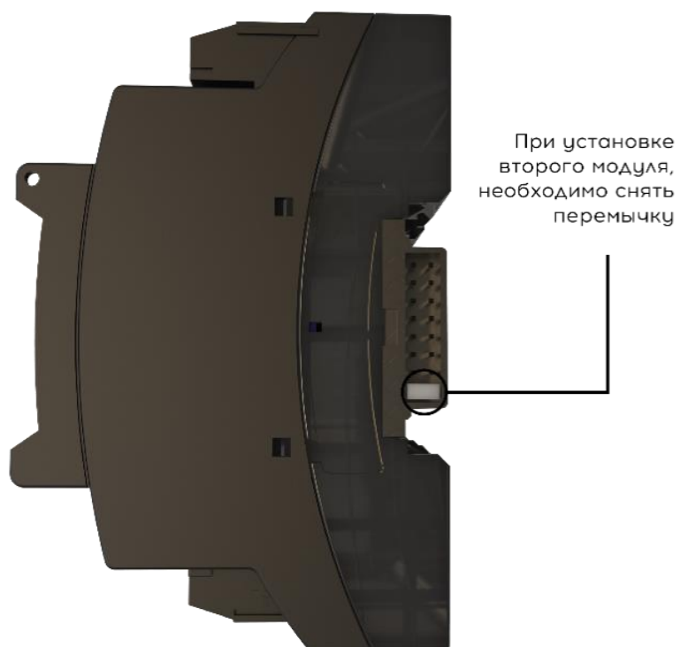
Рисунок 9.2 – Расположение перемычки в шинном соединителе
