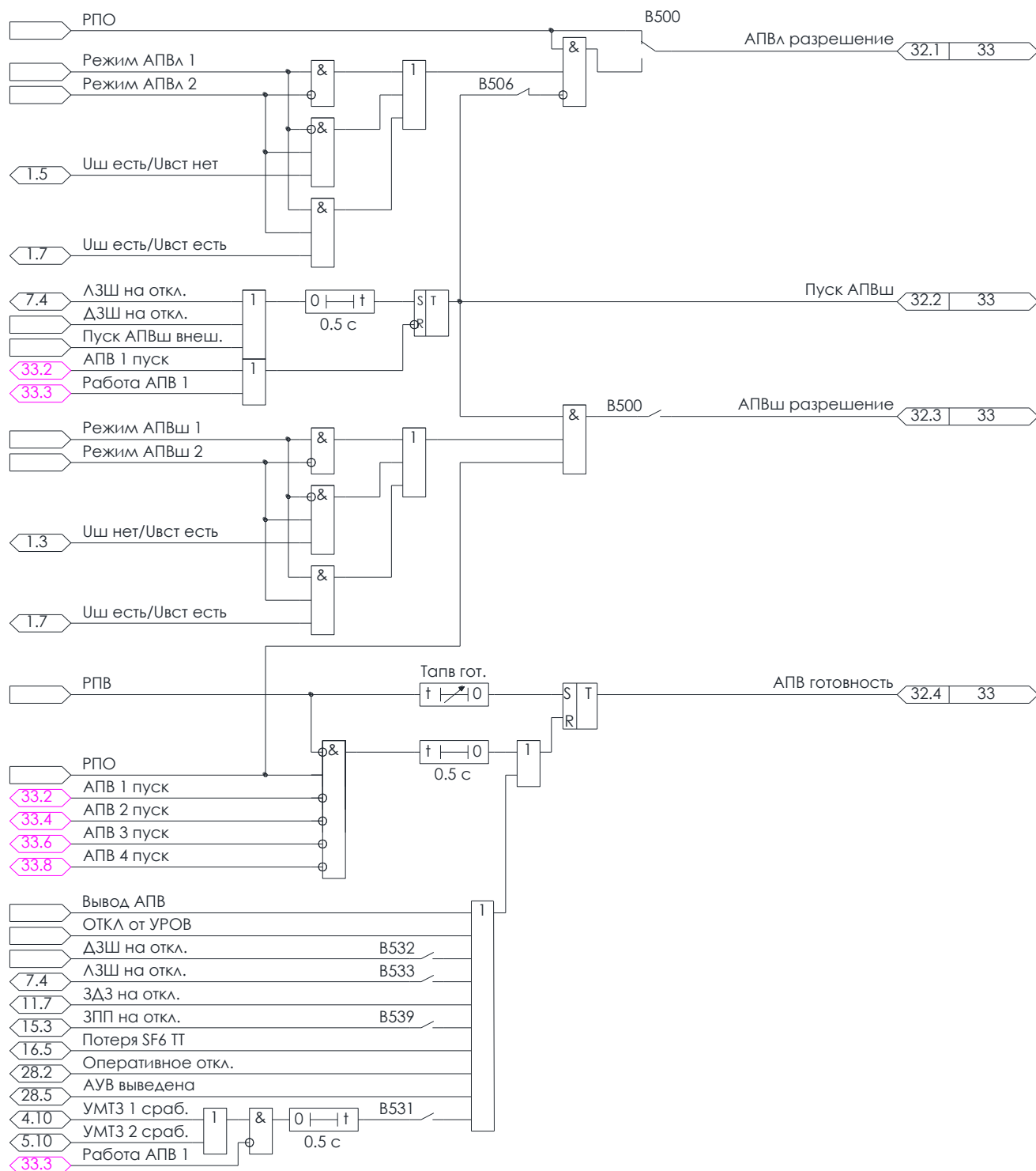
Рисунок 4.36 – Подготовка АПВ
