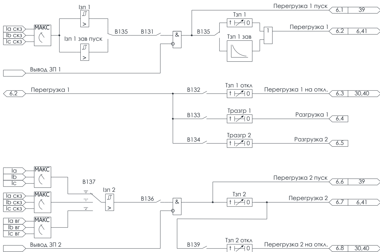
Рисунок 4.10 – Алгоритм ЗП
