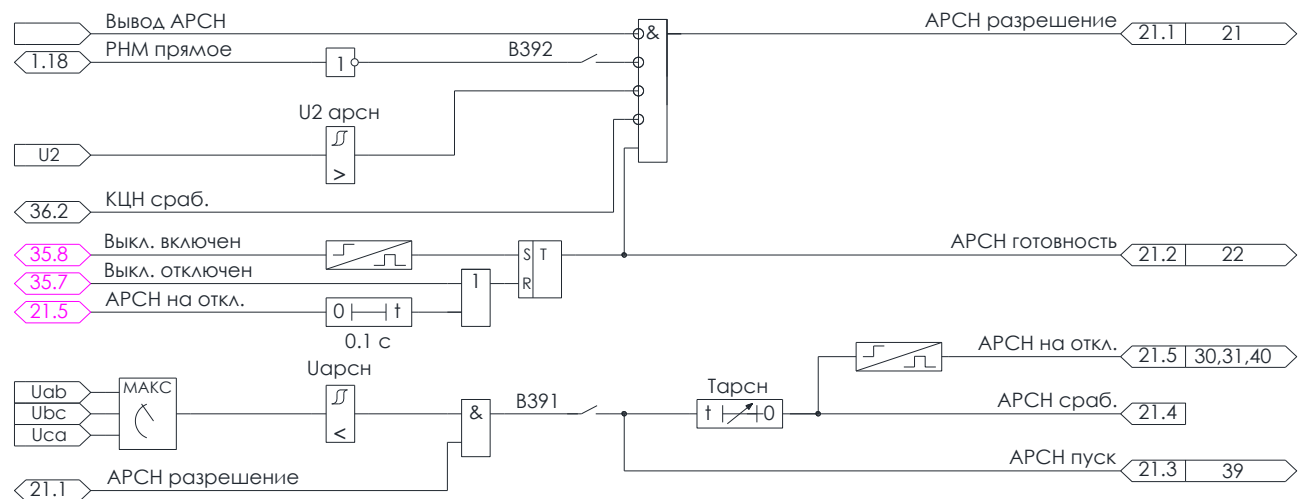
Рисунок 4.25 – Алгоритм АРСН
