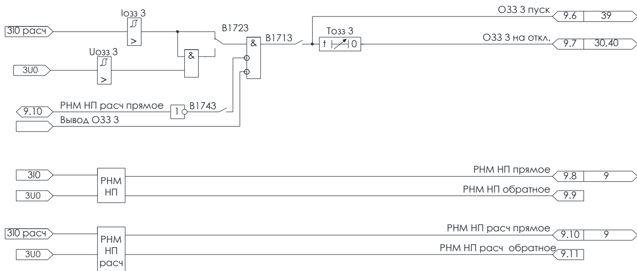
Рисунок 4.15 – Алгоритм третьей степени О33
