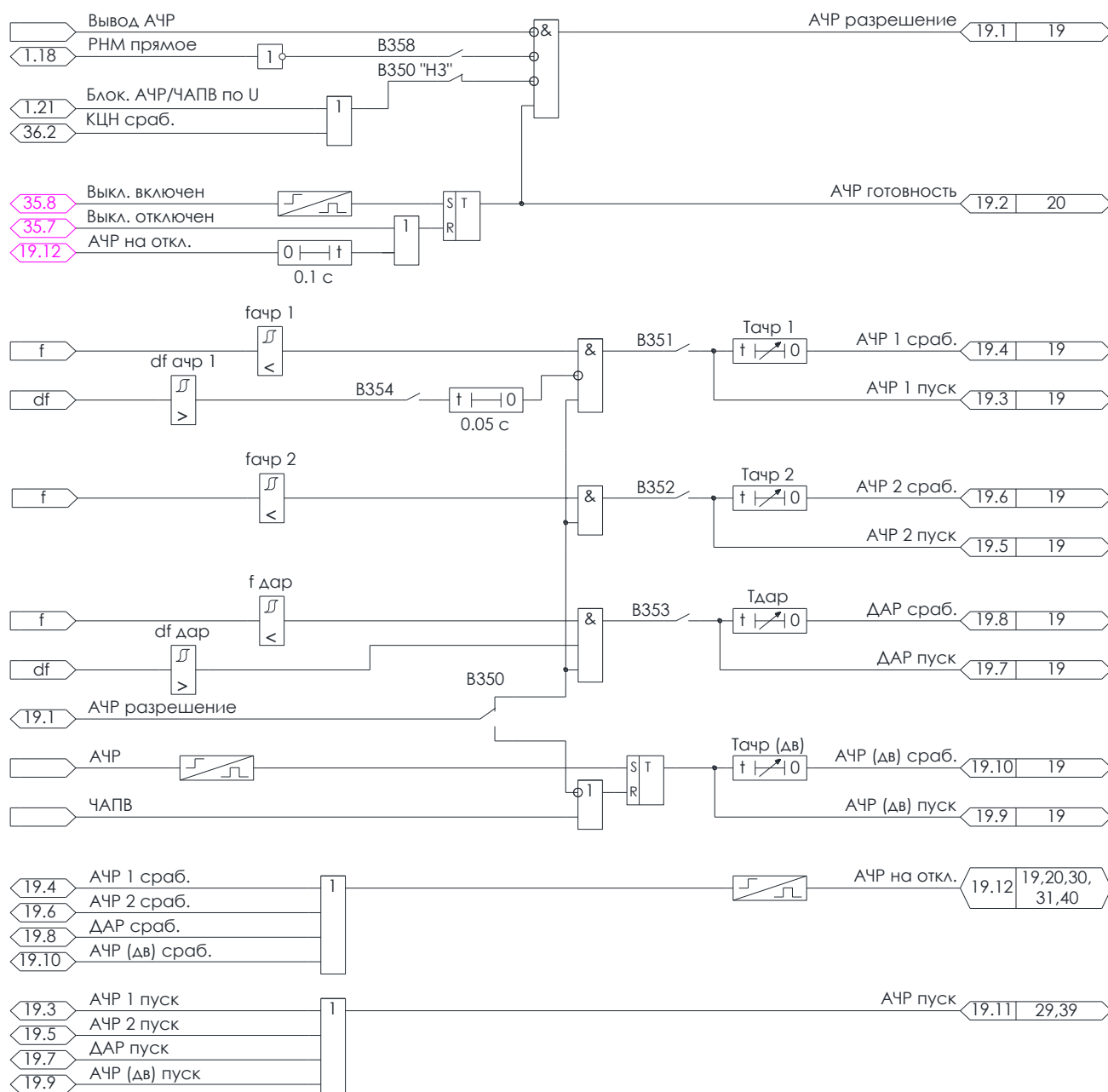
Рисунок 4.23 – Алгоритм АЧР
