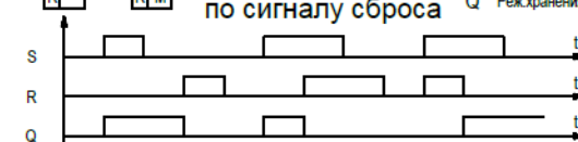
Триггер с приоритетом по сигналу сброса
