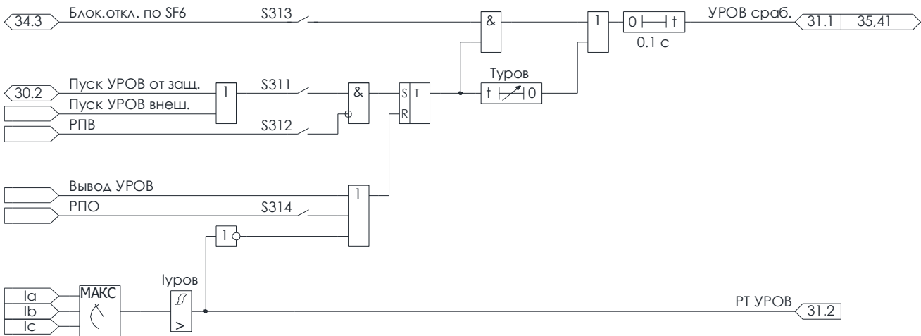
Рисунок 4.22 – Алгоритм УРОВ
