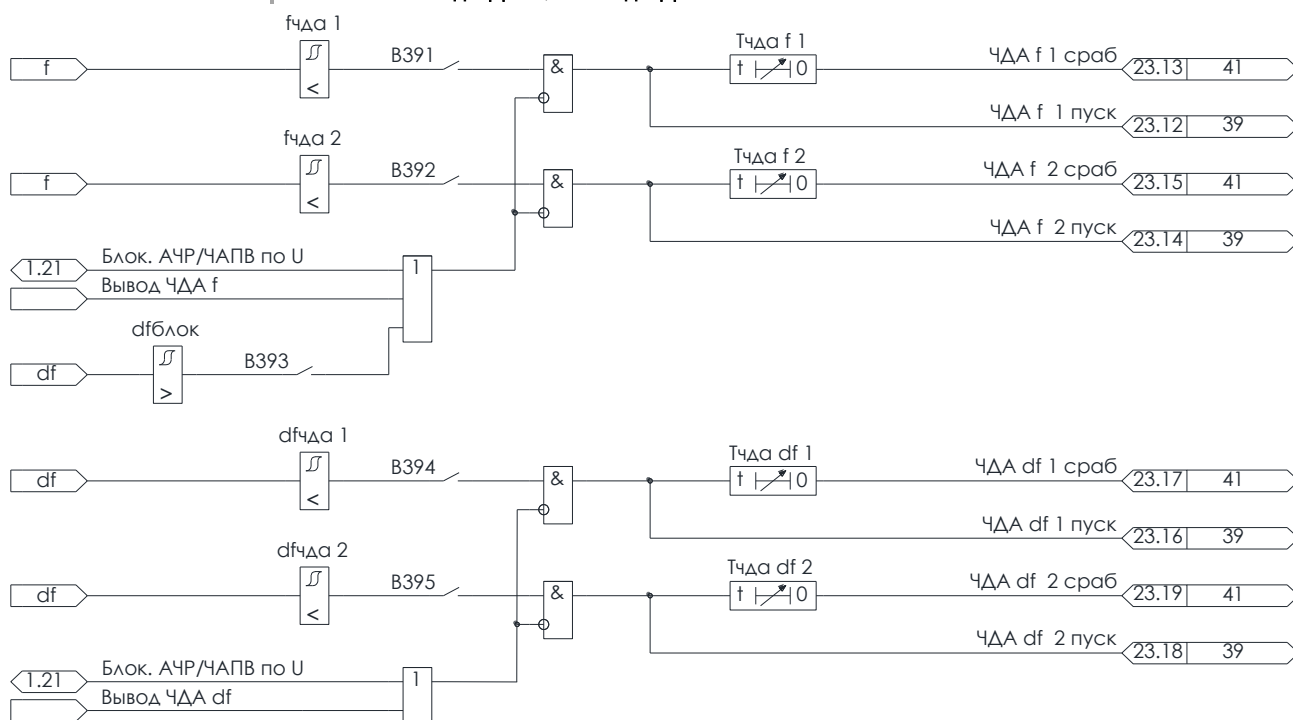
Рисунок 4.28 – Алгоритм АОПЧ
