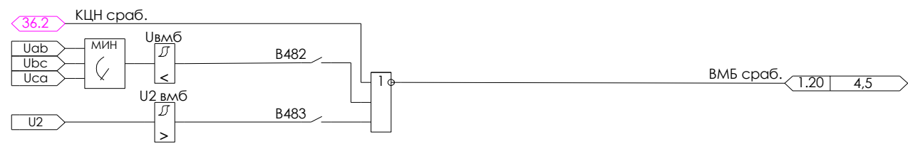
Рисунок 4.4 – Вольтметровая блокировка
