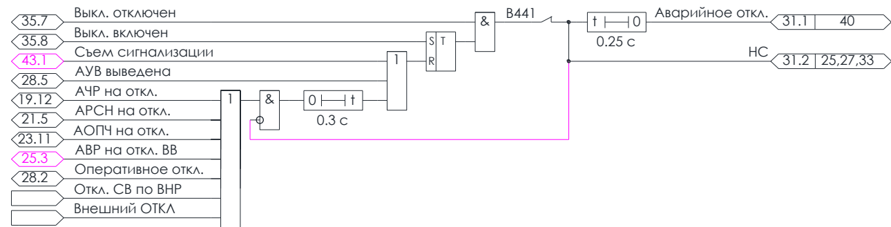
Рисунок 4.35 – Алгоритм аварийного отключения
