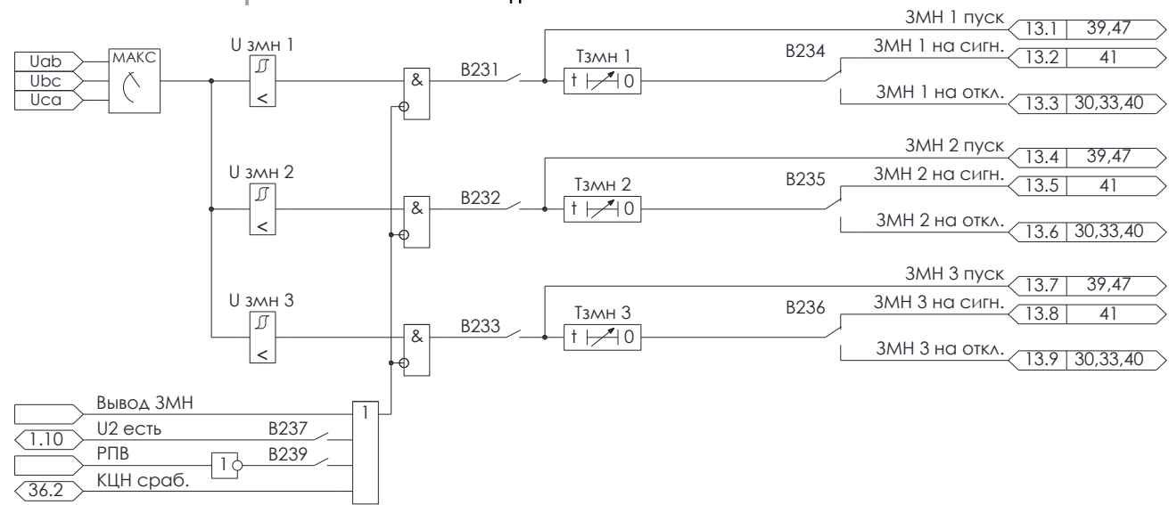
Рисунок 4.18 – Алгоритм ЗМН
