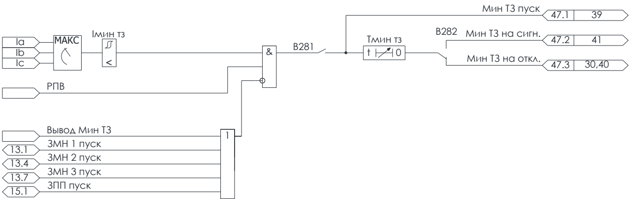
Рисунок 4.42 – Алгоритм МинТЗ
