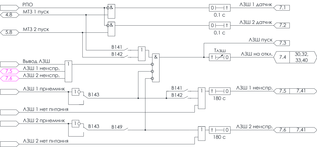
Рисунок 4.11 – Алгоритм ЛЗШ
