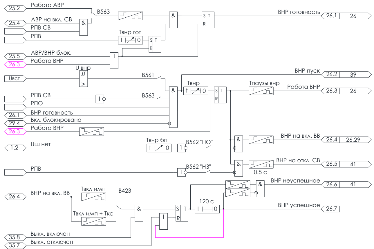
Рисунок 4.30 – Алгоритм ВНР
